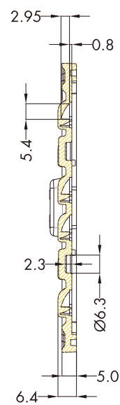
SECTION A-A
