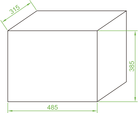
外盒Cardboard -485*315*385
